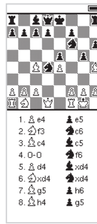
Рисунок 5. Отмена/список ходов.
