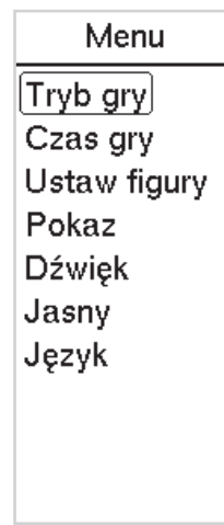
Fig 2. Menu.
