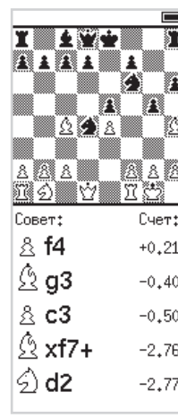
Рисунок 6. Подсказка.
