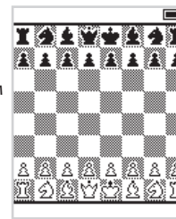
Рисунок 3. Подсветка клеткопозиции.
